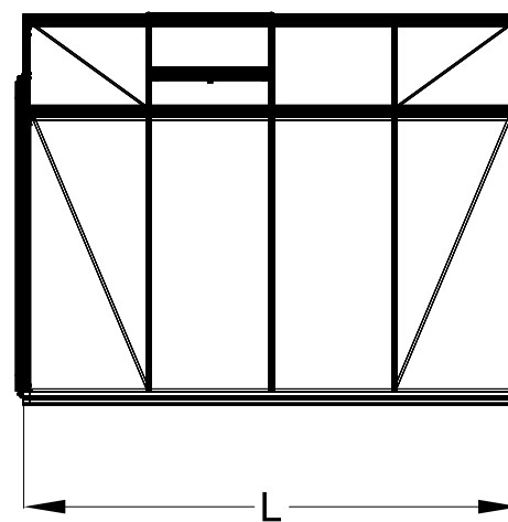
Right/leftview
